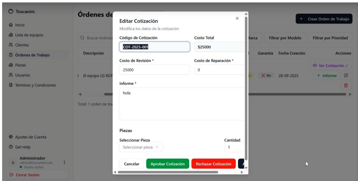
Figura 3.134 CU2.2.4 Estado distinto para No Reparable
