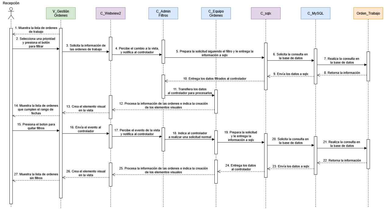
Figura 3.44 DDS Filtrando órdenes por Prioridad (Recepción)
