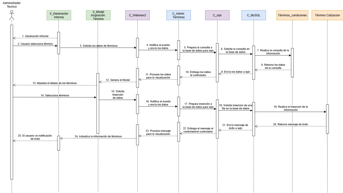
Figura 3.18 DDS Agregando términos y condiciones a documentos (Informe Técnico)
