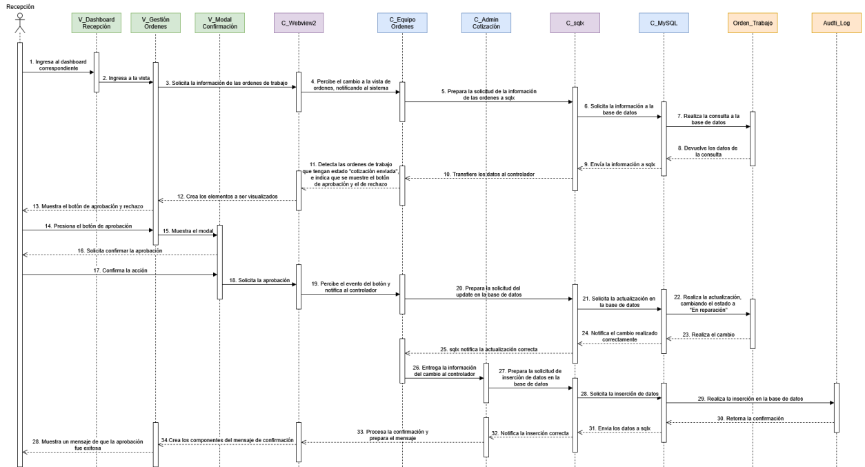
Figura 3.9 DDS Aprobando cotización de un equipo
