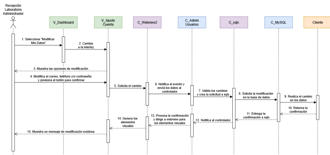
Figura 3.27 DDS Modificando datos personales de usuario
