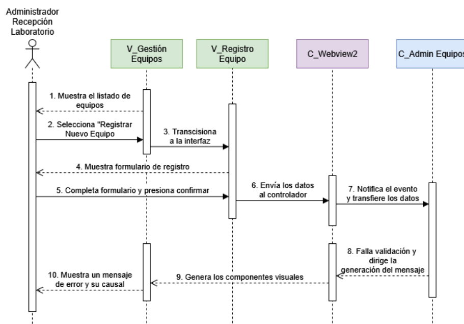
Figura 3.31 DDS Alternancia Registrando nuevo equipo en inventario
