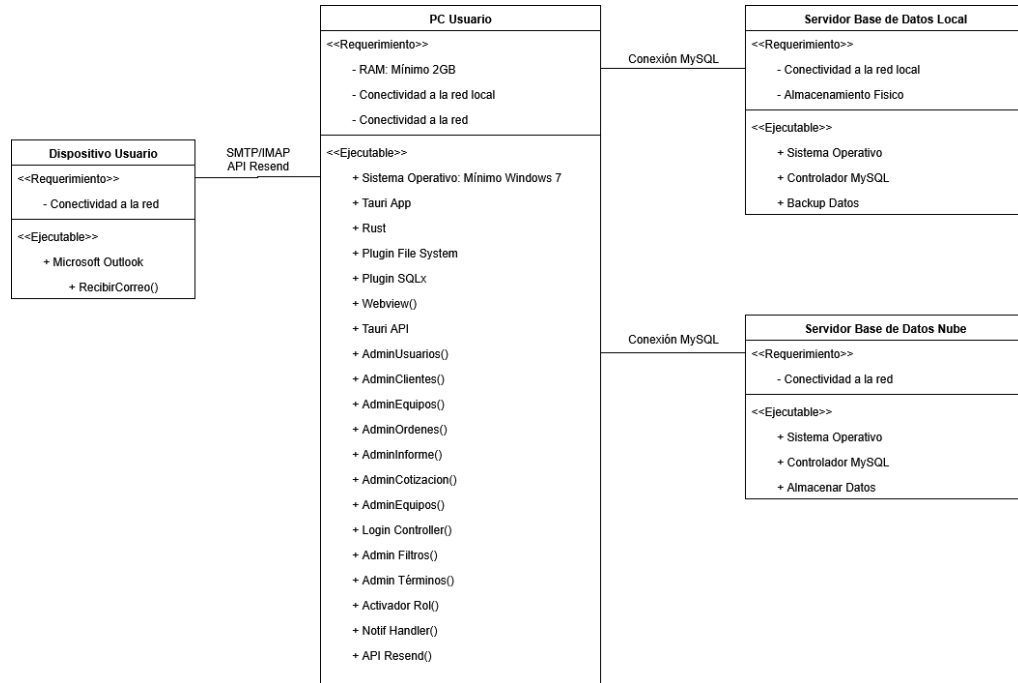
Figura 3.53 Diagrama de Despliegue del Sistema
