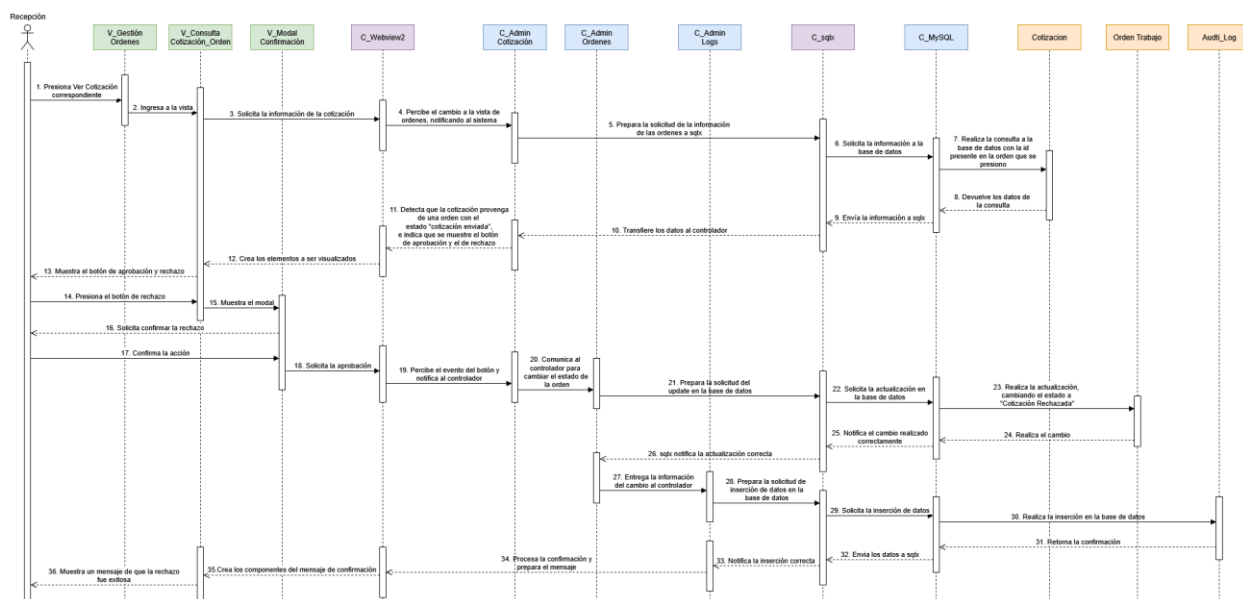
Figura 3.12 DDS Alternancia Rechazando cotización de un equipo
