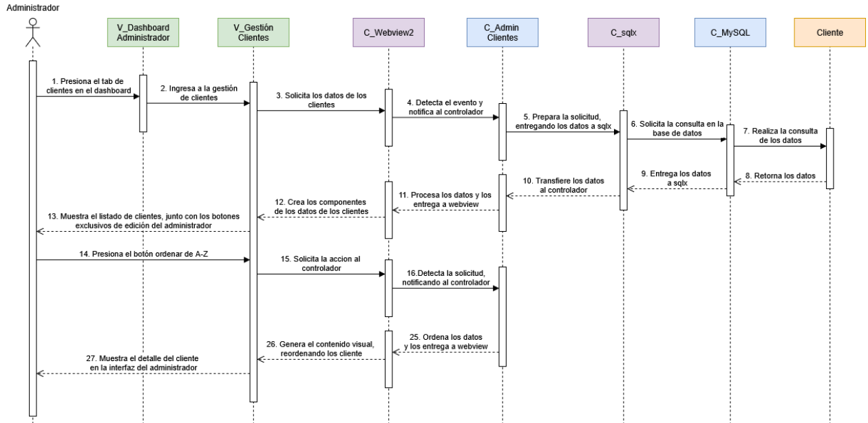
Figura 3.51 DDS Ordenando clientes alfabéticamente
