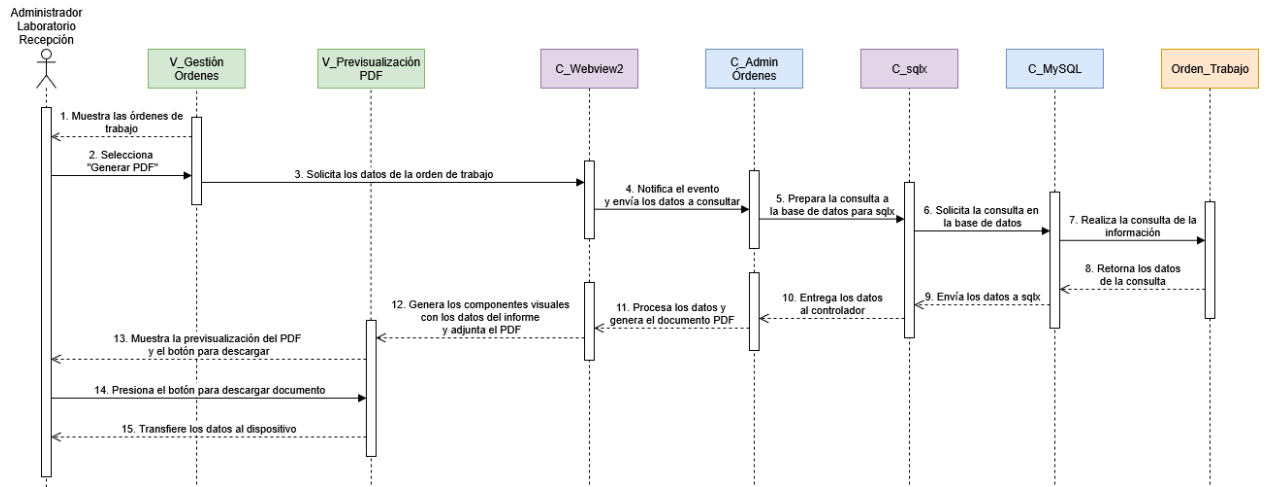
Figura 3.13 DDS Generando y visualizando documento en PDF
