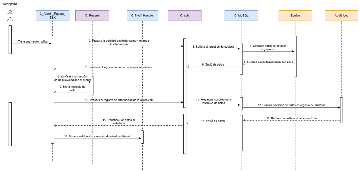
Figura 3.37 DDS Enviando correo de confirmación al cliente
