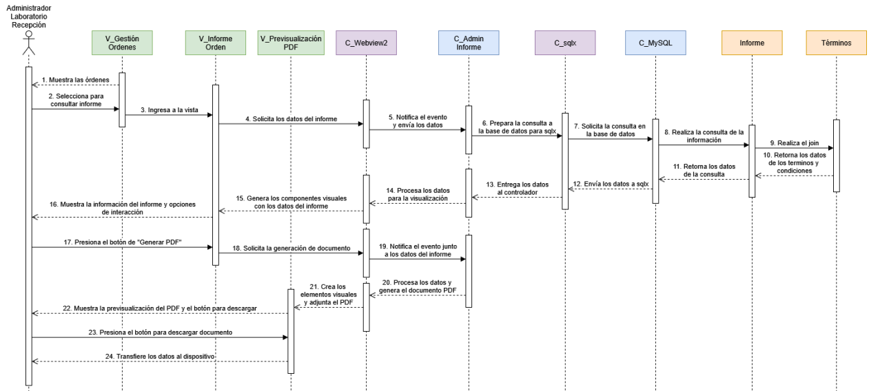
Figura 3.15 DDS Alternancia 2 Generando y visualizando documento en PDF
