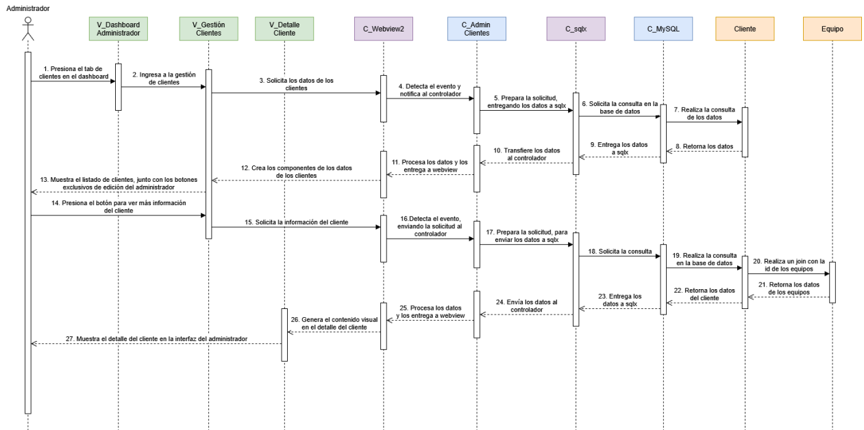
Figura 3.23 DDS Visualizar clientes registrados (Administrador)
