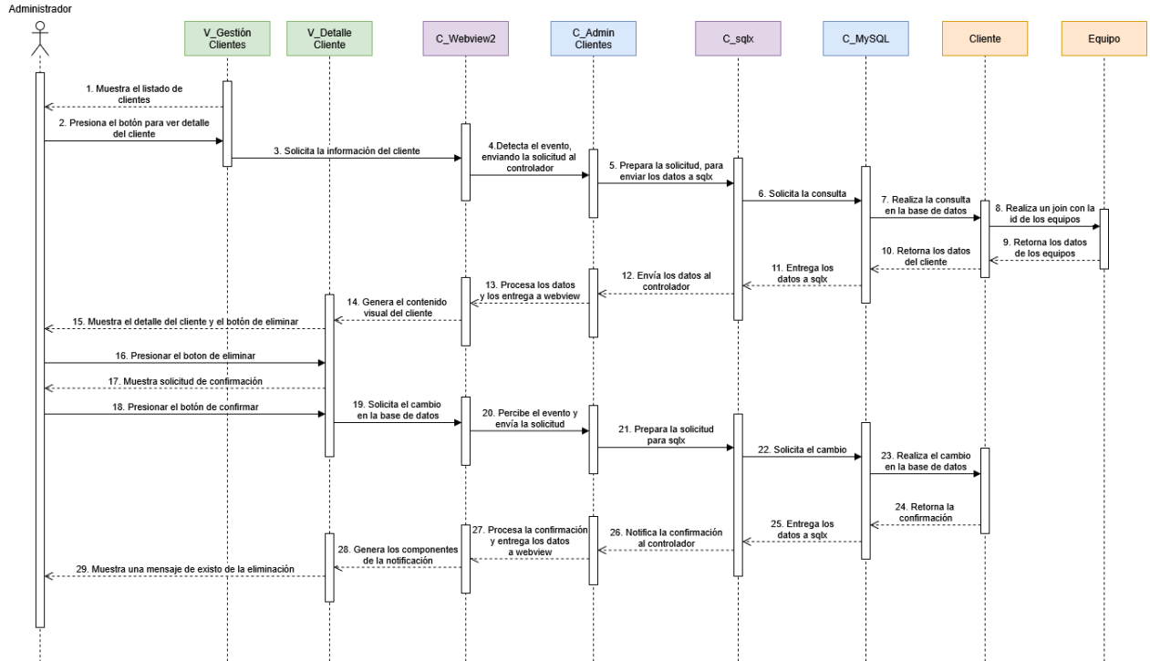
Figura 3.24 DDS Eliminando Clientes
