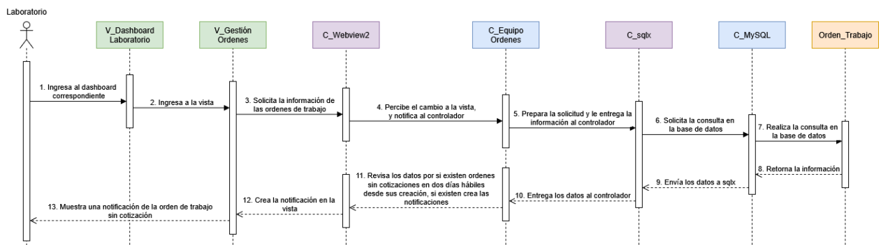
Figura 3.34 DDS Notificando por cotización no realizada
