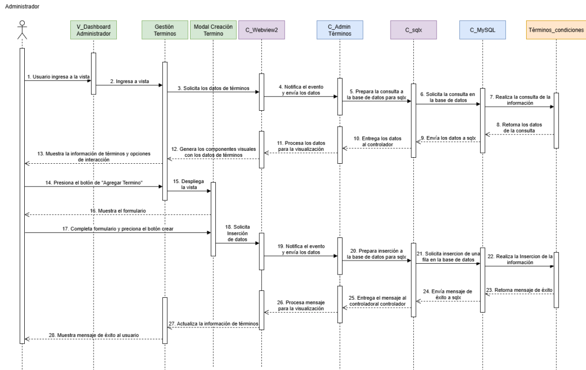
Figura 3.16 DDS Creando y gestionando términos y condiciones (Cotizaciones e Informes)
