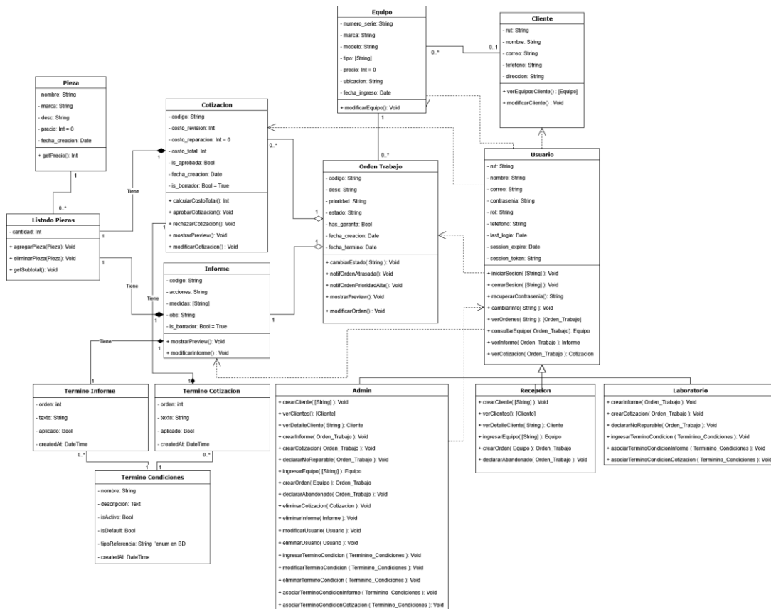
Figura 3.2 Diagrama de Clases de las entidades del sistema
