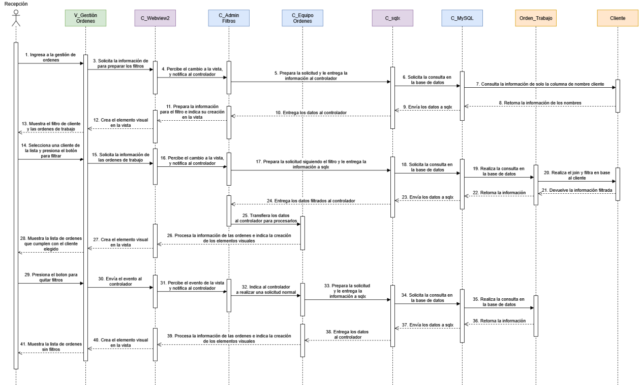
Figura 3.47 DDS Filtrando órdenes por Cliente (Recepción)
