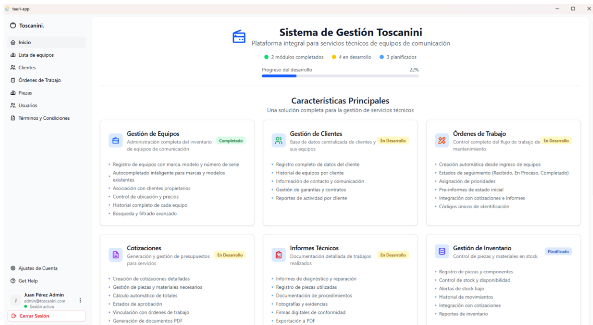
Figura 3.58 Dashboard Administrador
