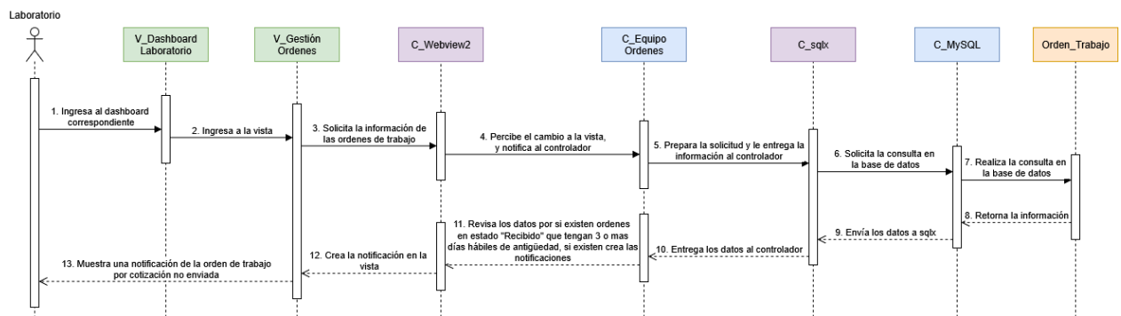
Figura 3.35 DDS Notificando por cotización no enviada
