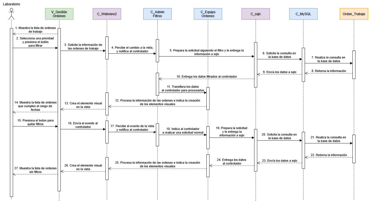
Figura 3.39 DDS Filtrando órdenes por Prioridad (Laboratorio)
