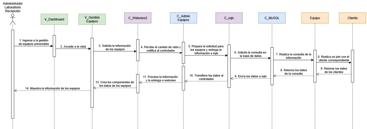
Figura 3.33 DDS Visualizar listado de equipos universales
