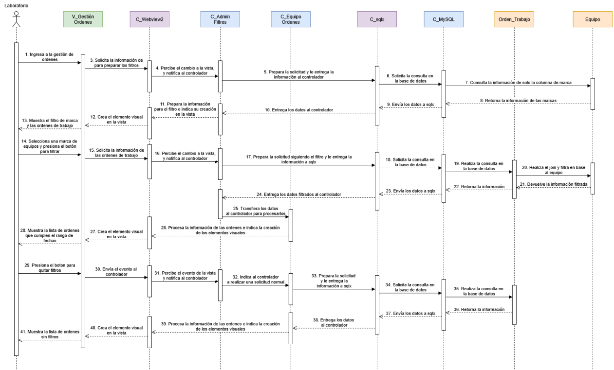
Figura 3.40 DDS Filtrando órdenes por Marca (Laboratorio)
